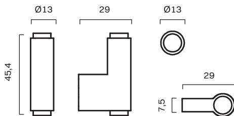
HOOK 45,4 mm
